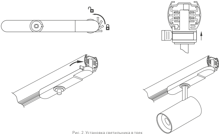
Рис. 2. Установка светильника в трек
