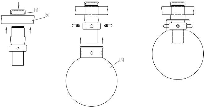
Рис. 2. Установка светильника
