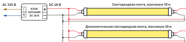
Схема 1. Подключение нескольких светодиодных лент «неон» с двух сторон
